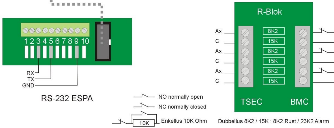
Aansturing ingangen
